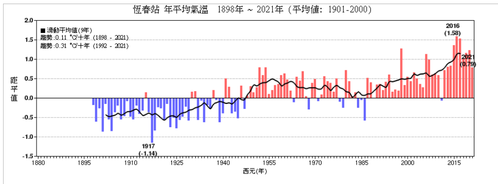
圖6，同圖2，但為1898-2021年恆春測站之溫度距平時間序列圖。
