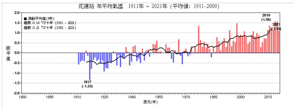
圖7，同圖2，但為1911-2021年花蓮測站之溫度距平時間序列圖。
