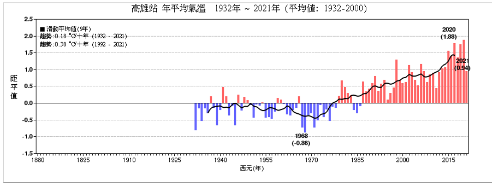
圖5，同圖2，但為1932-2021年高雄測站之溫度距平時間序列圖。
