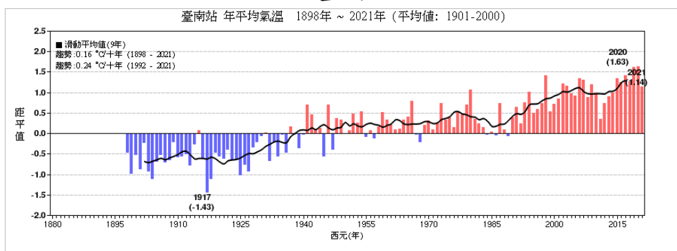
圖 4，同圖2，但為1898-2021年臺南測站之溫度距平時序圖。
