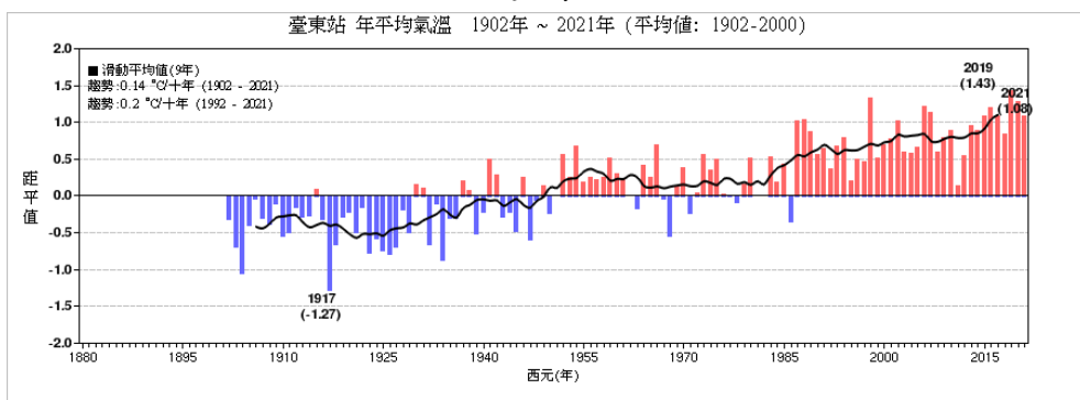
圖8，同圖2，但為1902-2021年臺東測站之溫度距平時間序列圖。
