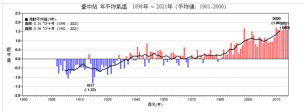
圖 3，同圖2，但為1898-2021年臺中測站之溫度距平時序圖。
