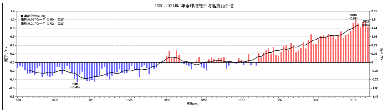
圖1. 1880-2021年全球溫度距平之時間序列圖，圖中紅/藍色長條分別表示正距平/負距平溫度，5年滑動平均為黑色實線，圖左上數值分別為百年及>近30年之上升趨勢值，單位為 ^{\circ}\text{C}/10\text{年} 。
